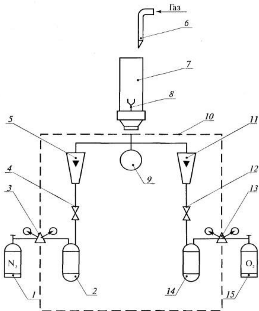
Рис. 1. Принципиальная схема лабораторной установки
