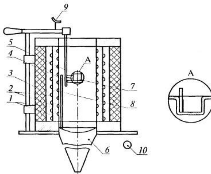
Рис. 1. Установка для определения температуры воспламеняемости конвейерных лент Порядок подготовки образцов
