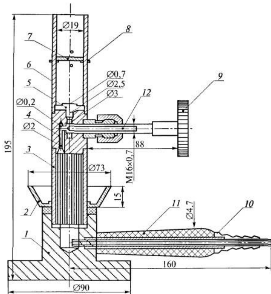
Рис. 2. Спиртовая горелка
