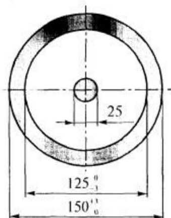
Рис. 2. Шаблон
