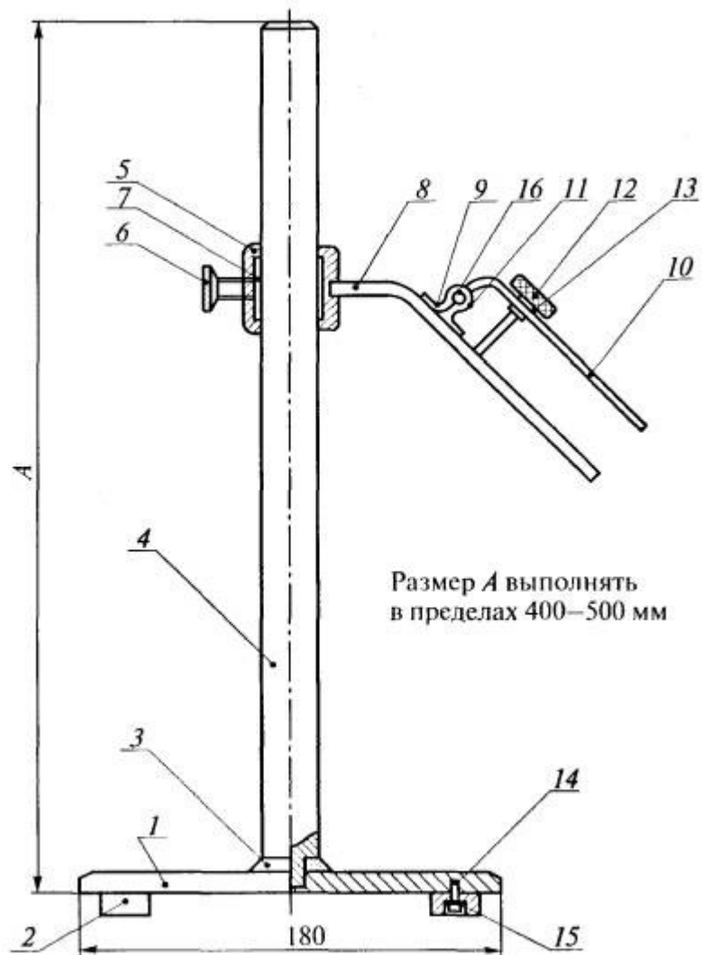
Рис. 3. Штатив с держателем
