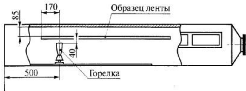
Рис. 1. Лабораторная модельная штольня типа А
