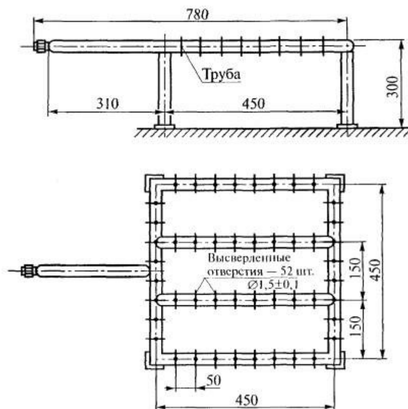
Рис. 2. Газовая (пропановая) горелка Проведение испытаний
