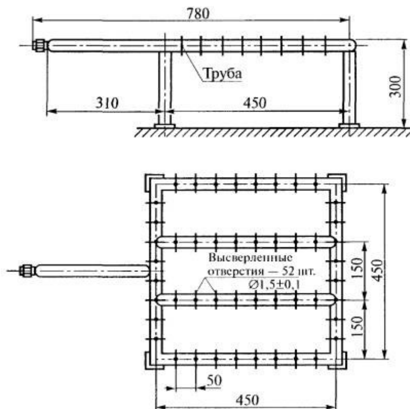
Рис. 8. Газовая горелка
