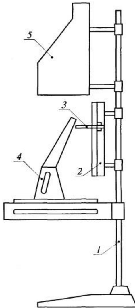
Рис. 1. Схема установки для определения индекса распространения пламени: 1 - стойка с держателем образца; 2 - электрическая радиационная панель; 3 - запальная горелка; 4 - термоэлектрический преобразователь для замера температуры продуктов горения; 5 - вытяжной зонт для сбора и удаления продуктов горения
