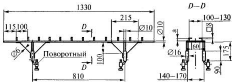
Рис. 4. Держатель образца
