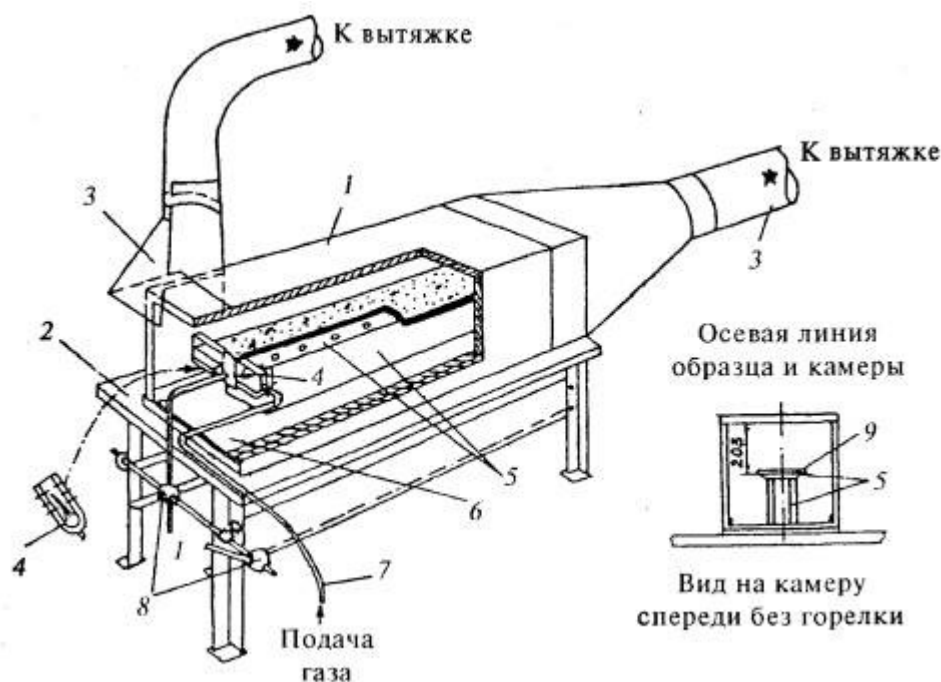
Рис. 6. Лабораторная модельная штольня типа Б
