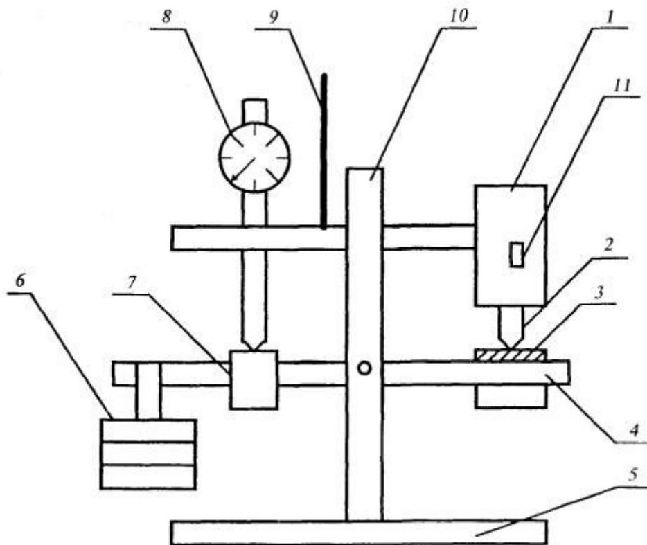
Рис. 1. Схема стенда для определения стойкости к прожиганию Порядок подготовки образцов
