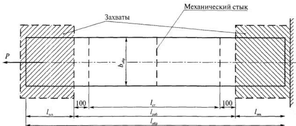
Рис. 1 Образец ленты
