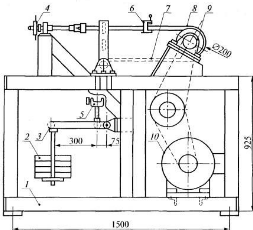
Рис. 1. Стенд для испытания лент на воспламеняемость при трении на барабане: 1 - станция; 2 - груз; 3 - рычаг; 4 - штурвал; 5 - нижний зажим; 6 - верхний зажим; 7 - образец ленты (сбегающая ветвь); 8 - образец ленты (набегающая ветвь); 9 - барабан; 10 - привод
