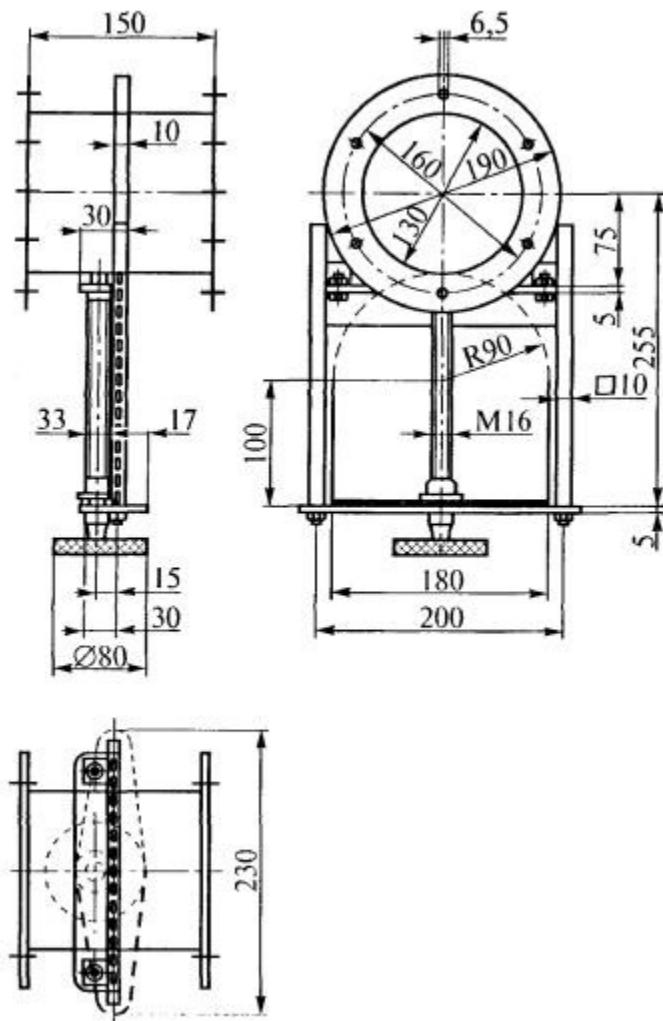
Рис. 3. Дроссельная заслонка
