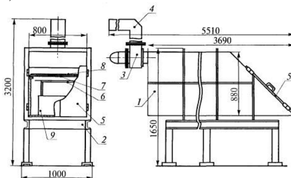
Рис. 7. Лабораторная модельная штольня типа В:
