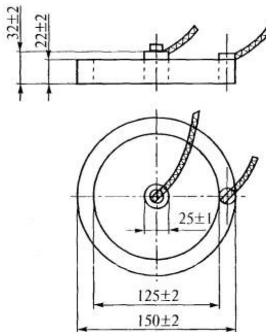
Рис. 1. Схема установки электродов
