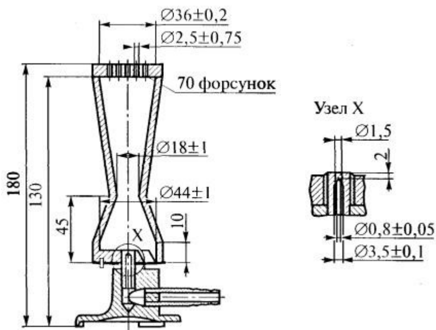
Рис. 5. Газовая горелка
